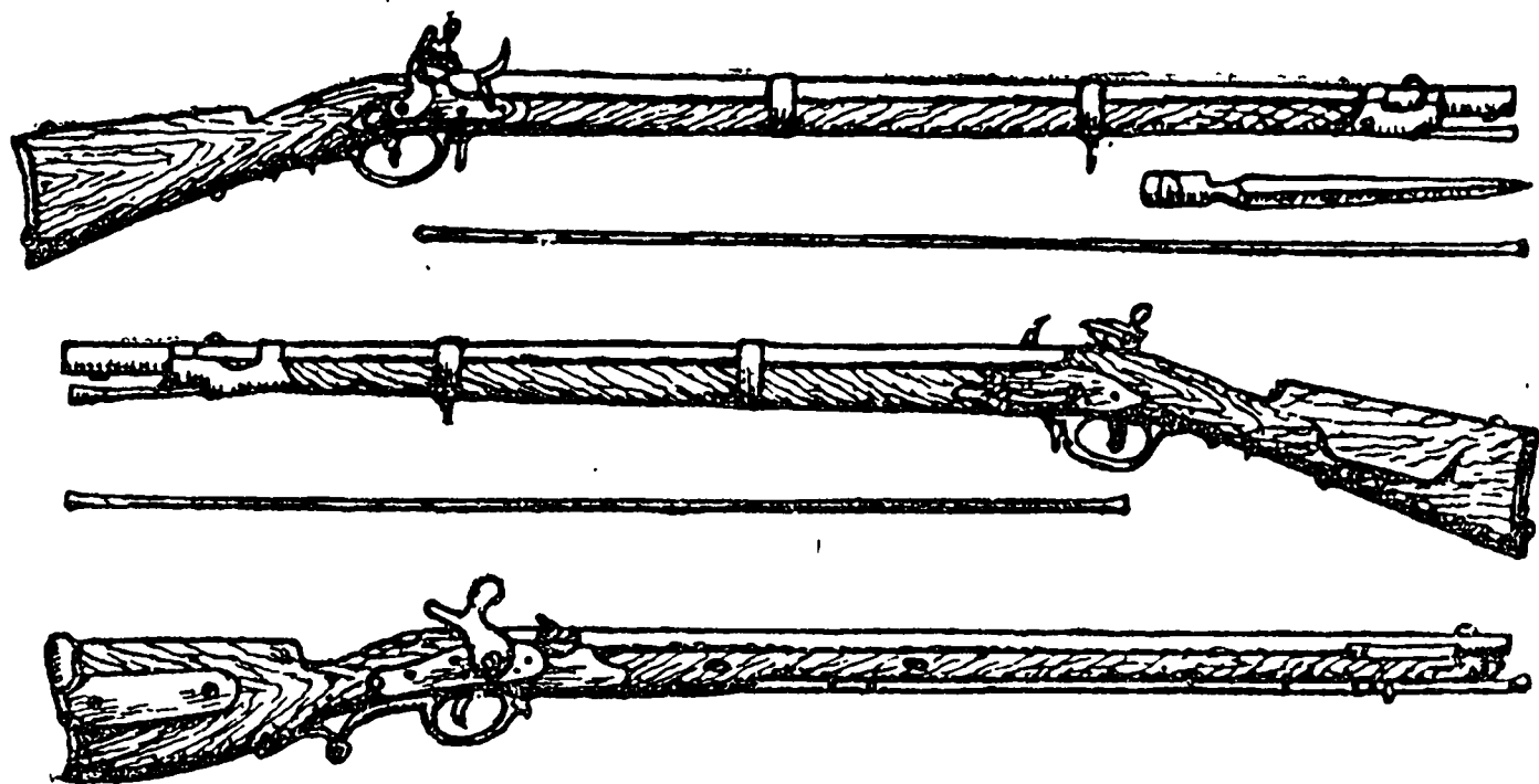
Кремневые пехотные ружья образца 1828 г. (Сверху вниз: драгунское, кирасирское и штуцер.)
